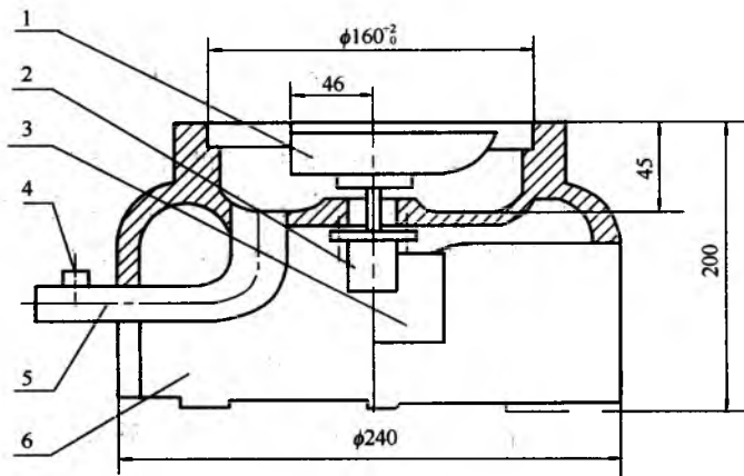
图 A. 3. 6 筛座示意图
