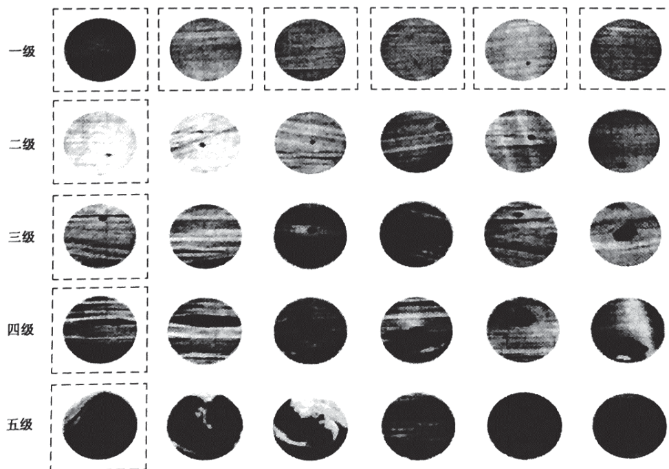
图 E.2 碳分散体分布图
