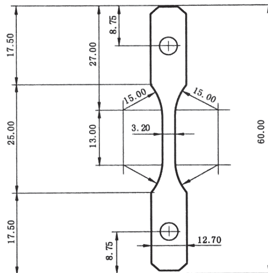
图 D.2 试样的尺寸图
