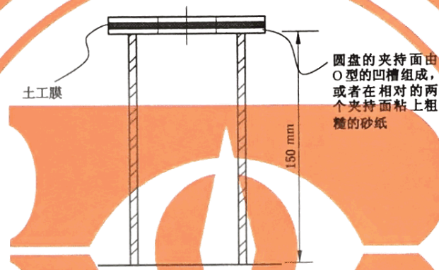
图 C.2 试验安装示意图(未按比例)
