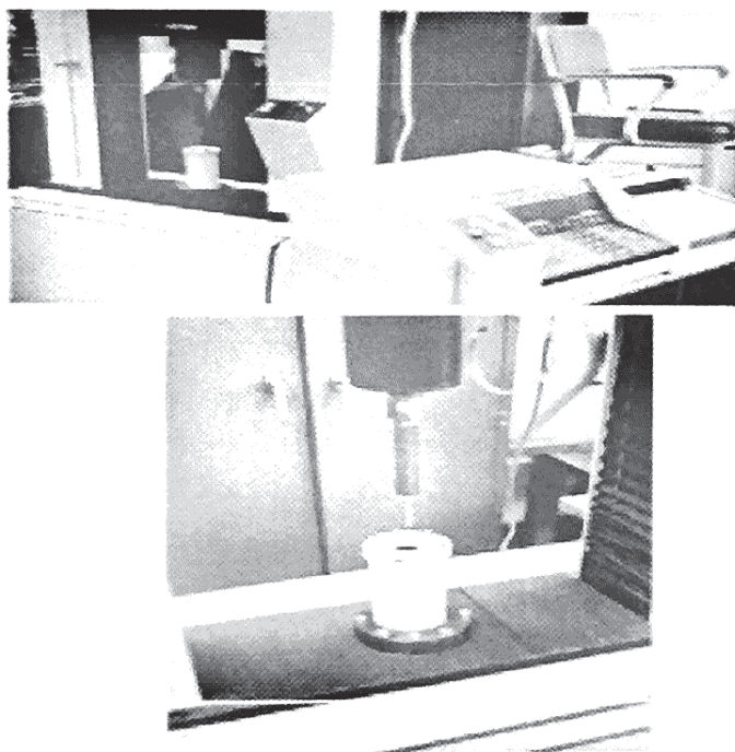
图 C.1 试验装置安装与固定的照片
