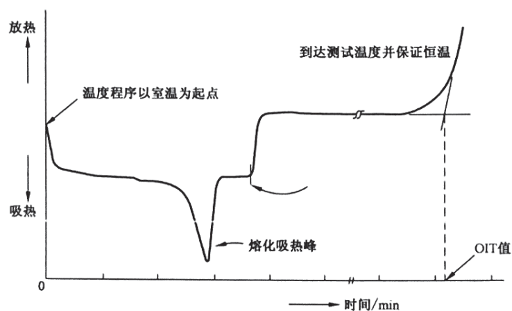
图 F.1 试验温度曲线图
