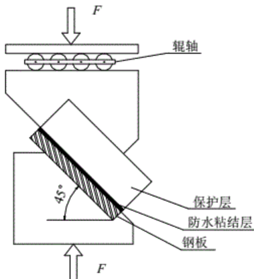
图 C.2.3 剪切强度试验方法示意图
