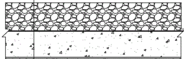
图 3-2 钢桥面铺装组合设计示例一
