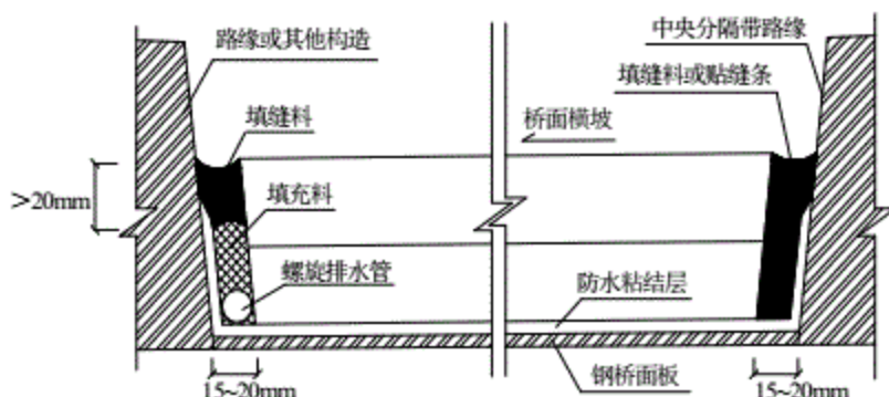
图 F.0.1-2 边缘排水处理细节
