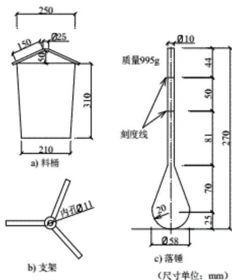
图 G.2.1 刘埃尔流动性试验设备
