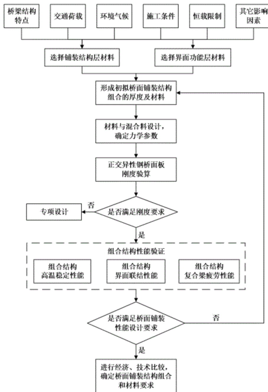
图 3-1 钢桥面铺装结构设计流程
