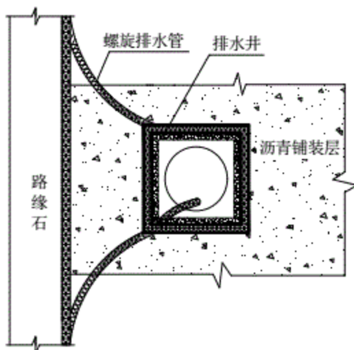
图 F.0.1-1 桥面铺装边部接缝构造
