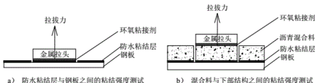
图 B.1.1 粘结强度试验方法示意图
