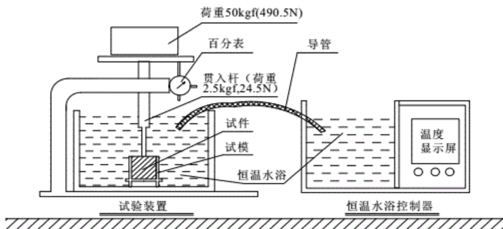
图 J.2.2 贯入度试验仪器
