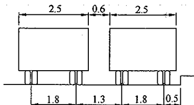
(6) 汽车荷载的横向布置
