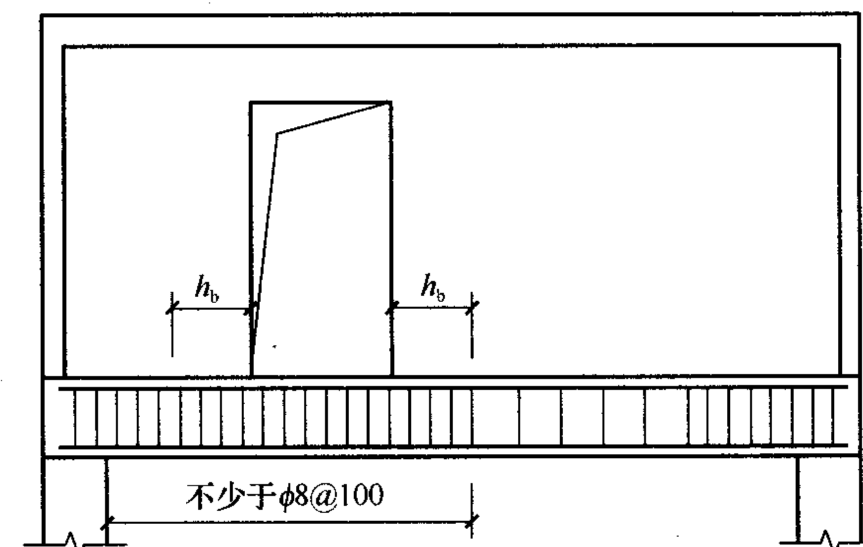
图 7.3.12 偏开洞时托梁箍筋加密区
