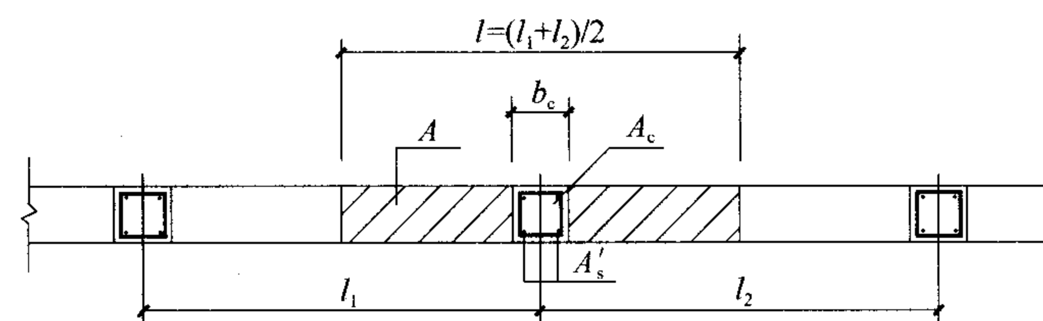
图 8.2.7 砖砌体和构造柱组合墙截面
