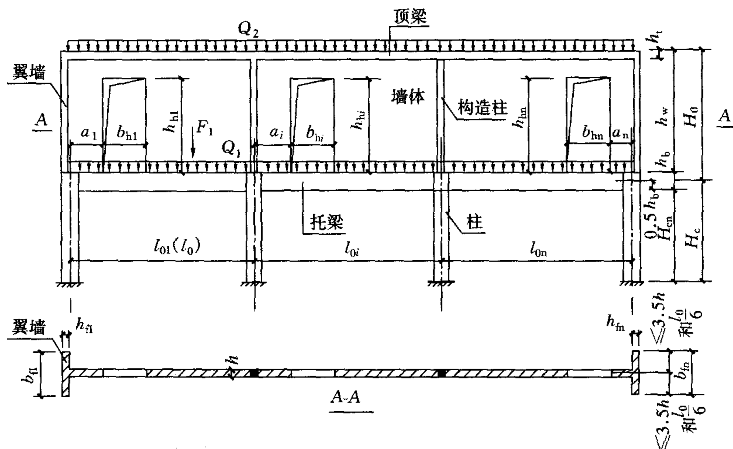
图 7.3.3 墙梁计算简图
