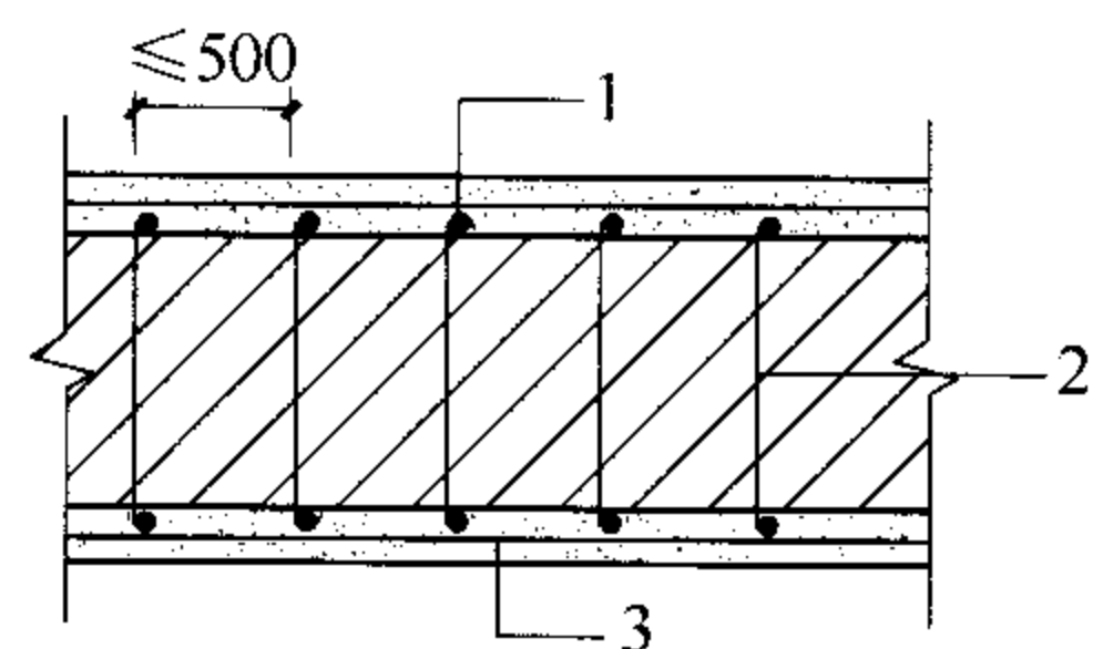
图 8.2.6 混凝土或砂浆 面层组合墙
