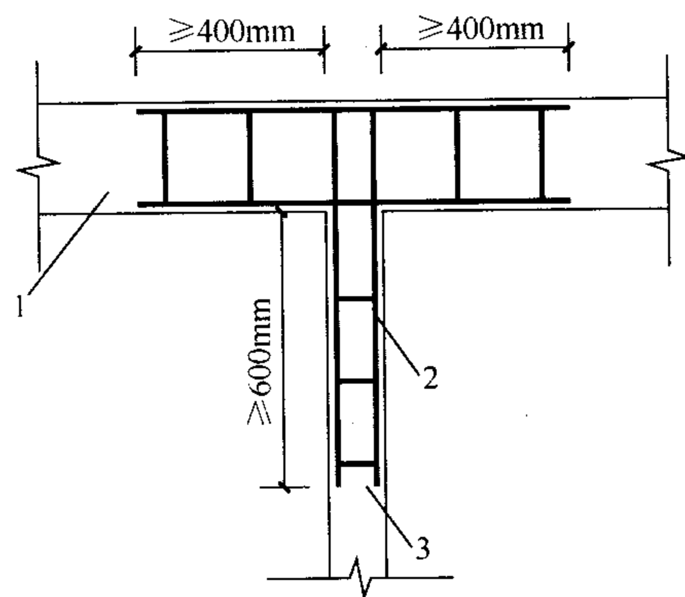
图 6.2.11 砌块墙与后砌隔墙交接处钢筋网片
