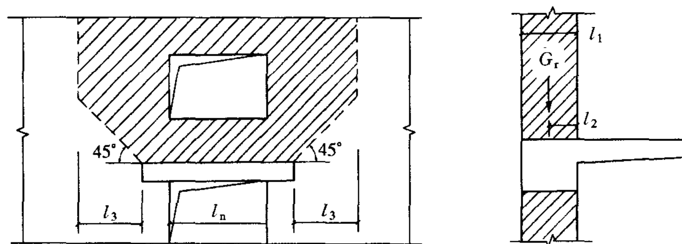
图 7.4.7 雨篷的抗倾覆荷载
