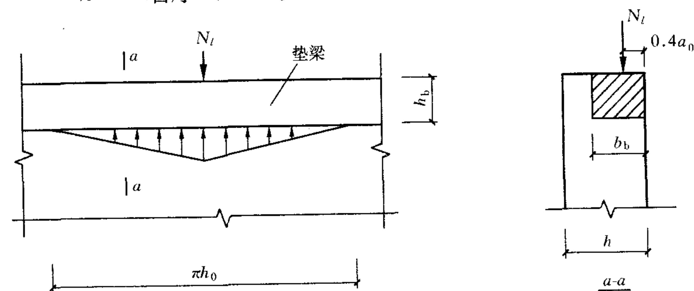
图 5.2.6 垫梁局部受压
