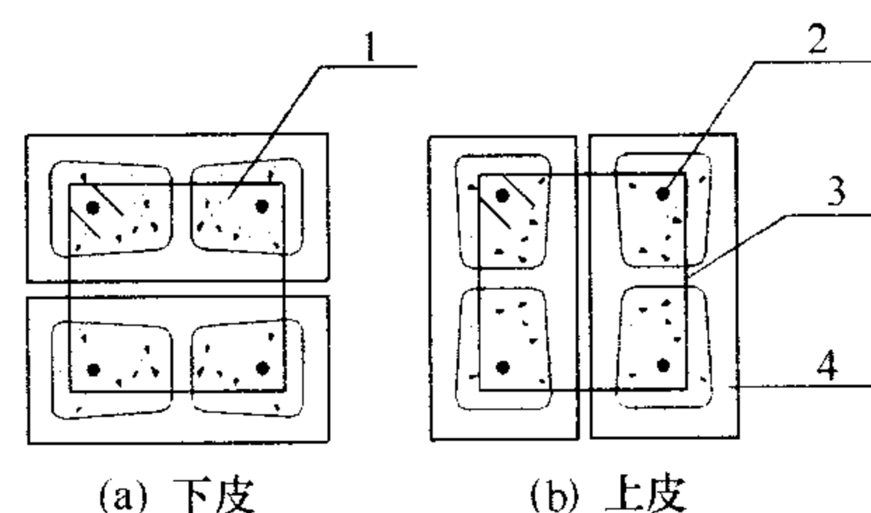
图 9.4.13 配筋砌块砌体柱截面示意 1—灌孔混凝土；2—钢筋；3—箍筋；4—砌块
