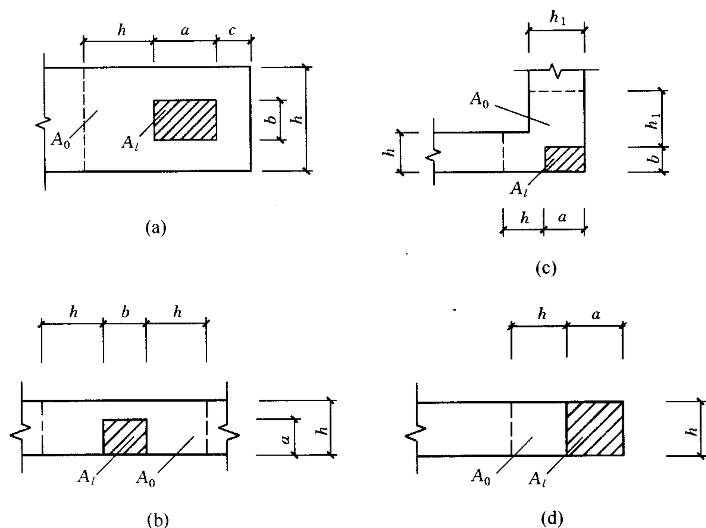
图 5.2.2 影响局部抗压强度的面积 A_0
