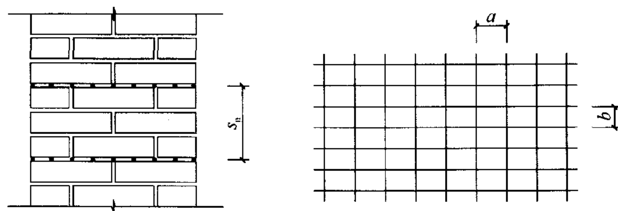
图 8.1.2 网状配筋砖砌体
