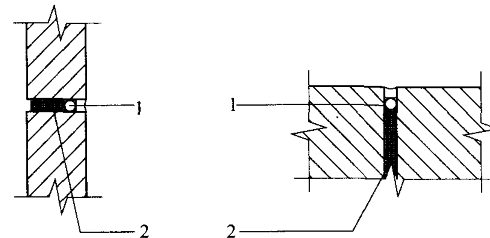
图 6.5.7 控制缝构造
