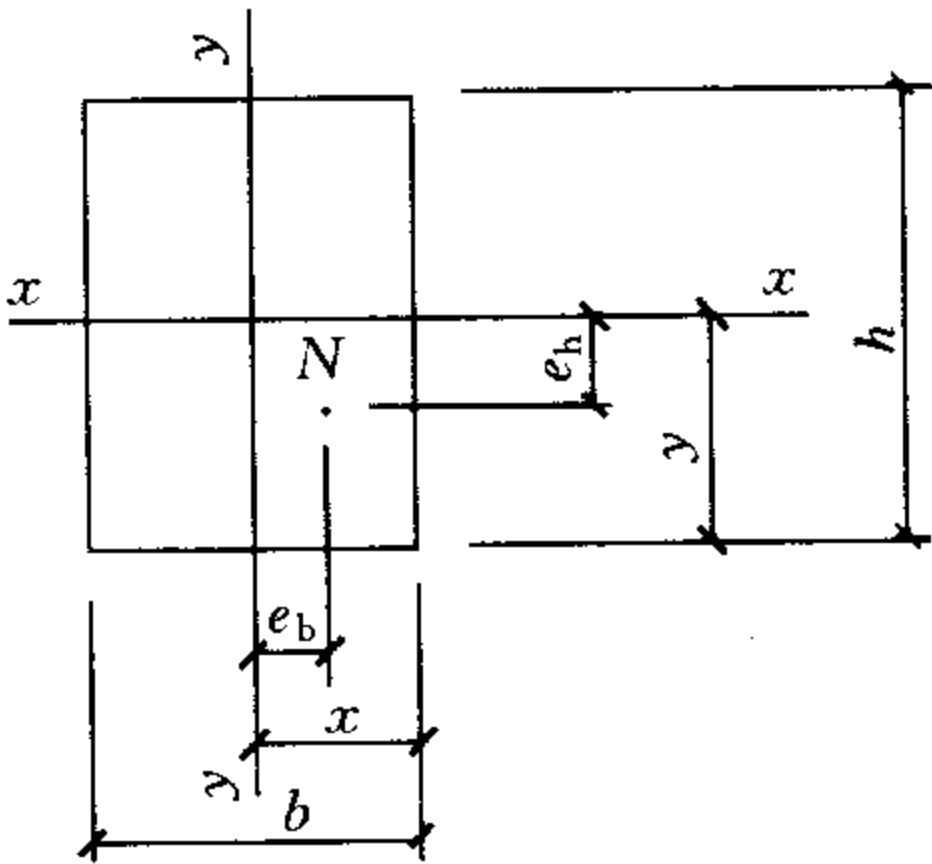
图 D.0.3 双向偏心受压
