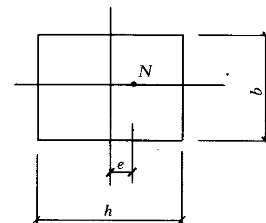
图 D.0.1 单向偏心受压
