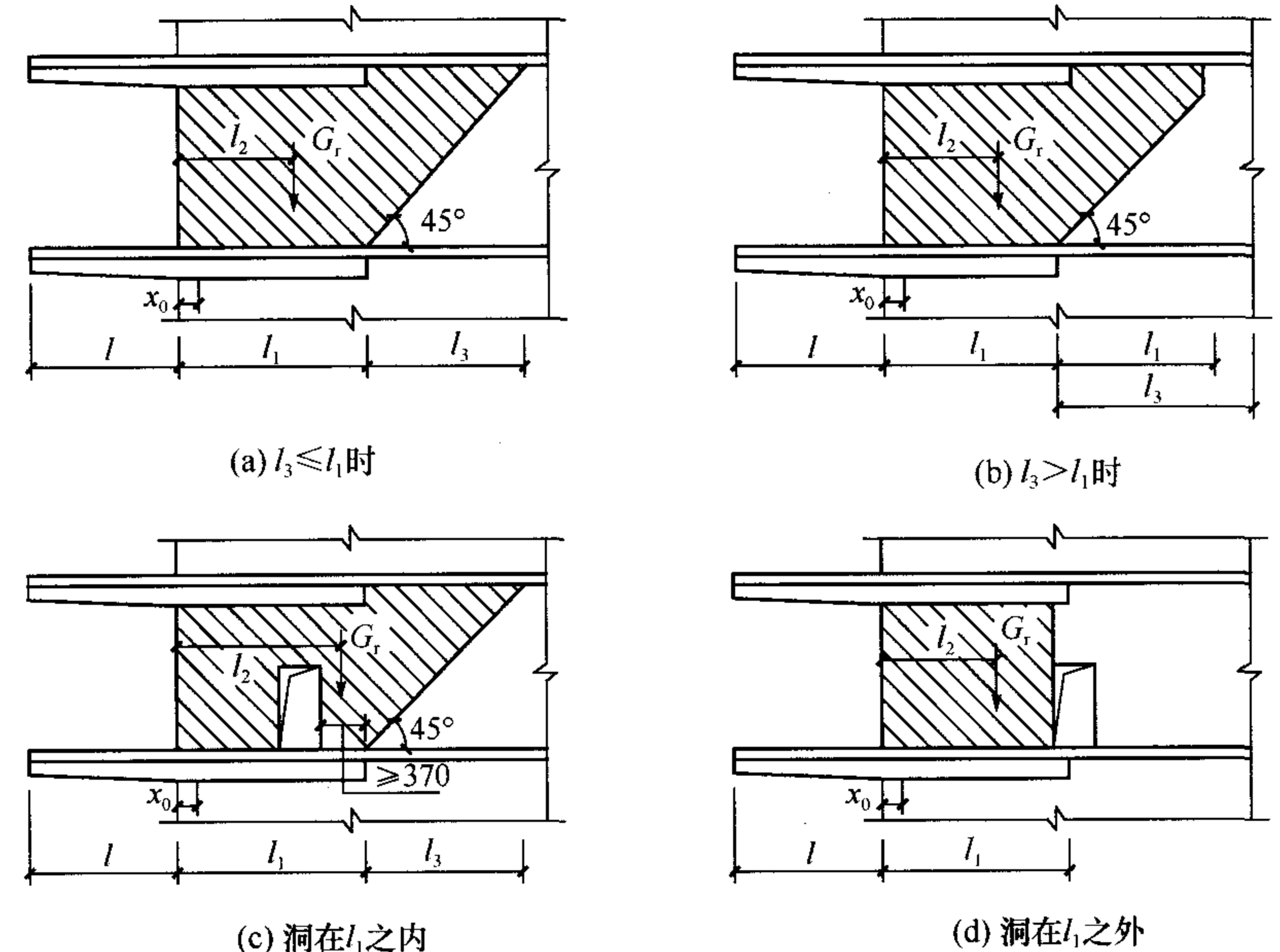
图 7.4.3 挑梁的抗倾覆荷载
