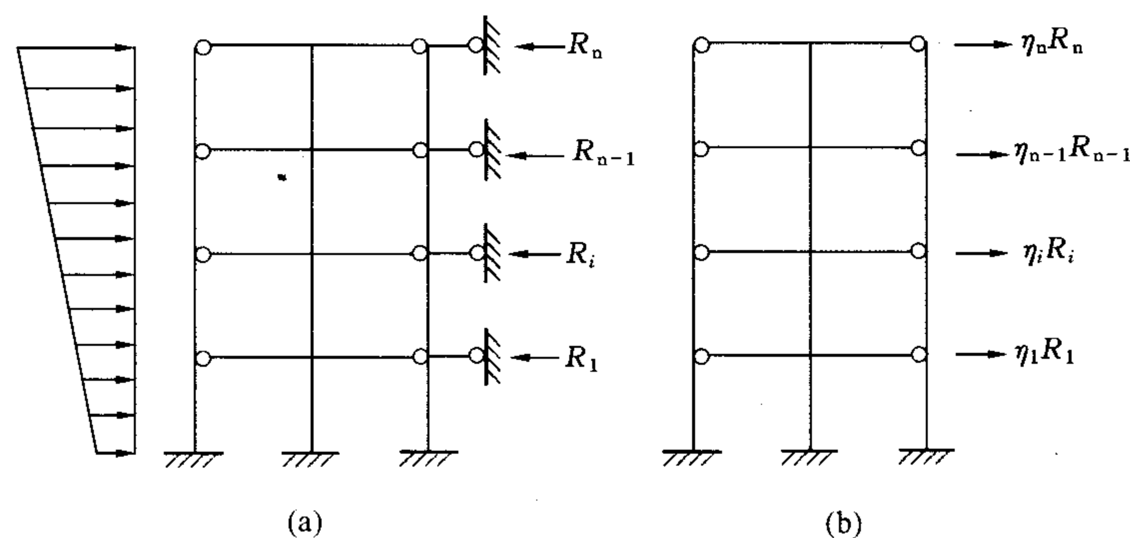
图 C.0.1 刚弹性方案房屋的静力计算简图
