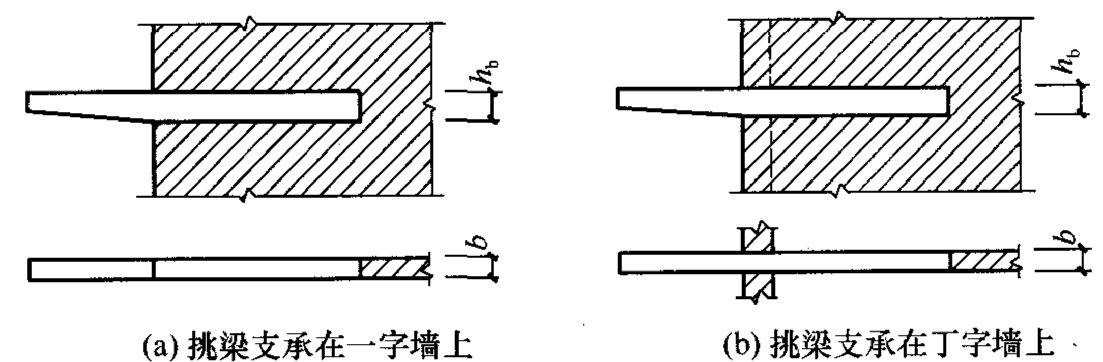
图 7.4.4 挑梁下砌体局部受压
