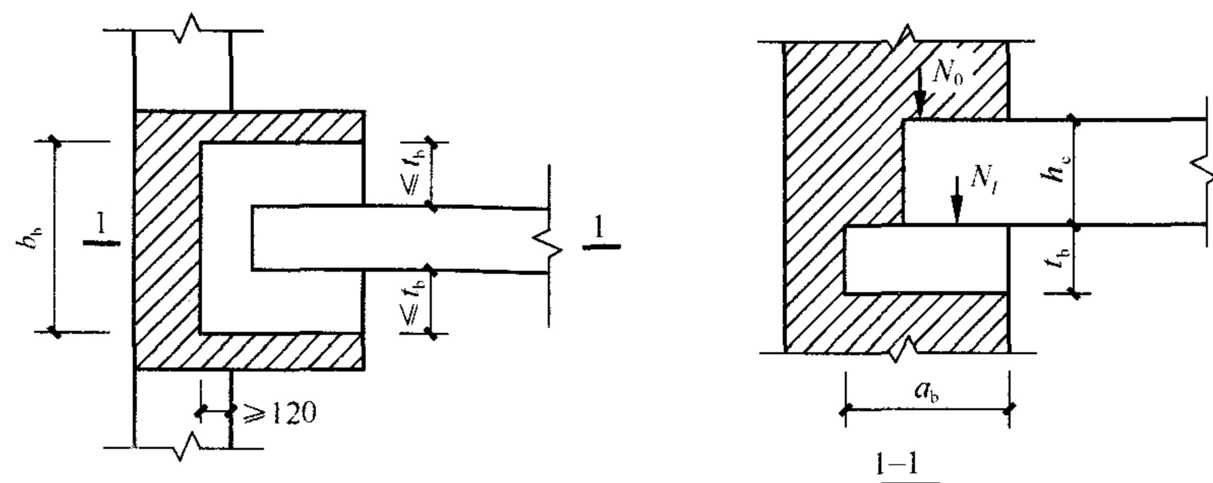
图 5.2.5 壁柱上设有垫块时梁端局部受压
