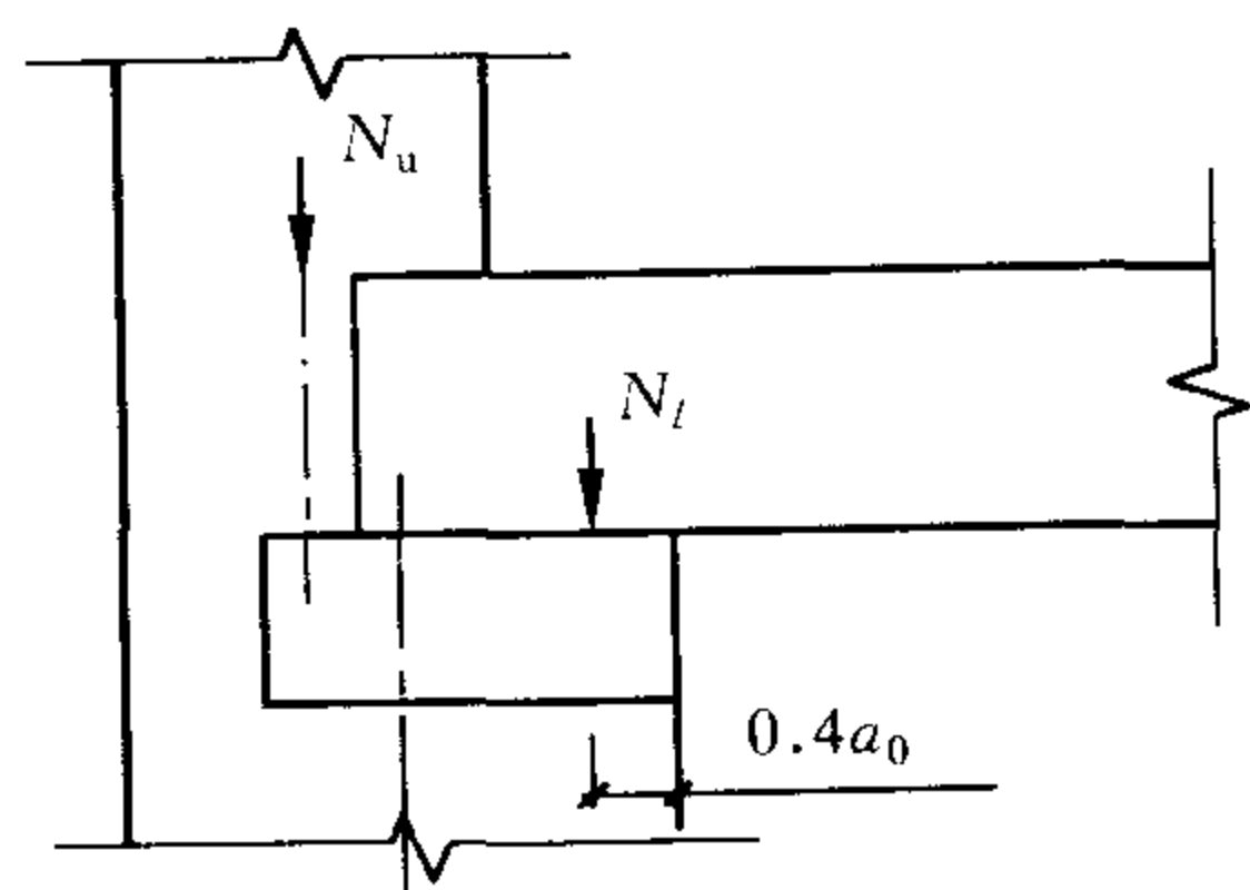
图 4.2.5 梁端支承压力位置
