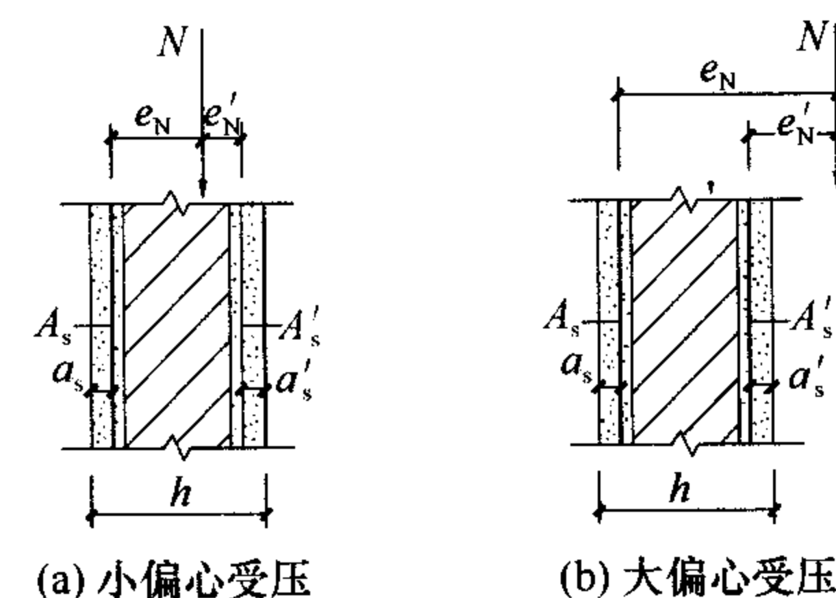
图 8.2.4 组合砖砌体偏心受压构件
