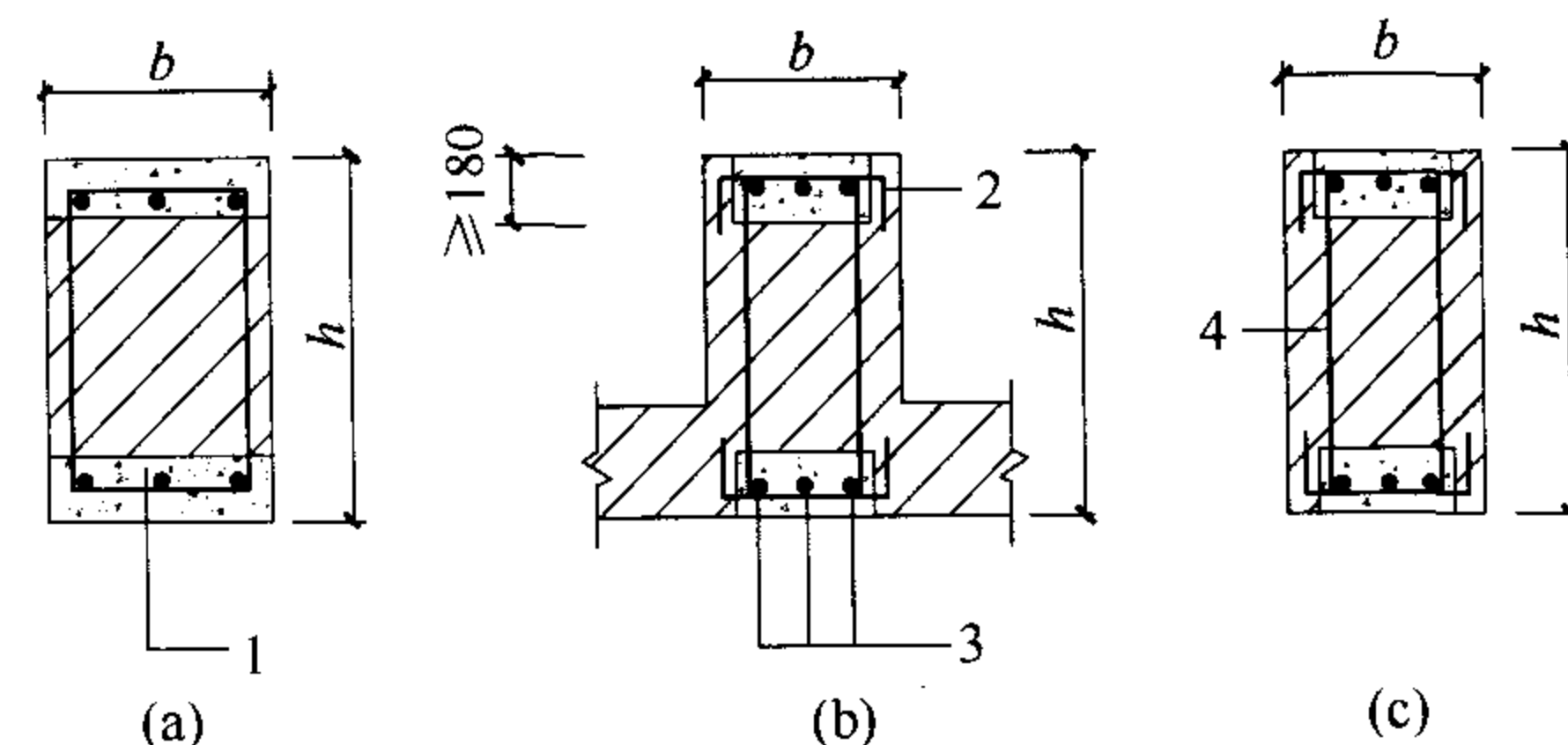
图 8.2.1 组合砖砌体构件截面
